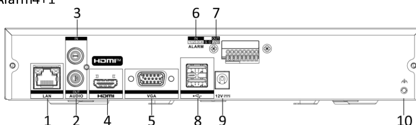
DS-7608NI-Q1(E)/Alarm4+1
