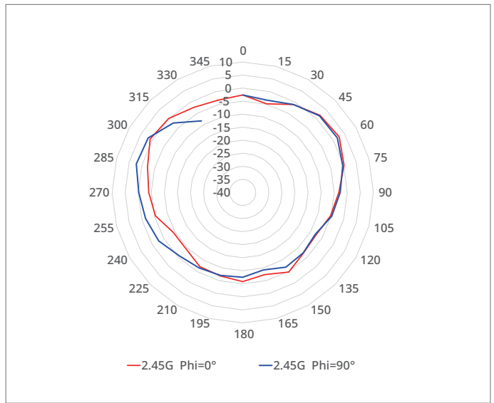
2.4 GHz (ANT1, 2, 3, 4)
