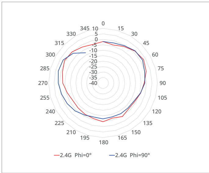
2.4 GHz (ANT1, 2, 3, 4)
