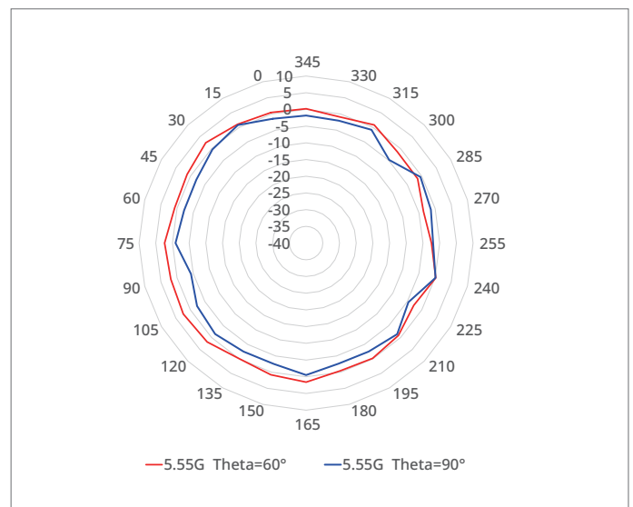
5.5 GHz (ANT1, 2, 3, 4)
